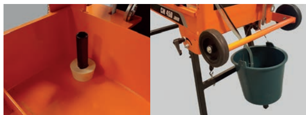
VÍZLEERESZTŐ RENDSZER
